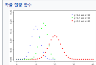
이항분포
