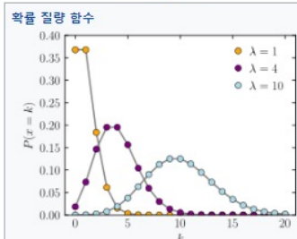
푸아송 분포
